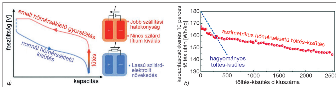
35. ábra. Aszimmetrikus hőmérsékletű töltés-fogyasztás ciklusának karakterisztikája és hatása a garantált működési ciklusszáma [5]
