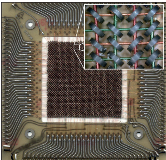
2. ábra. A ferritgyűrűs írható-olvasható memóriaegység felépítése [2]
