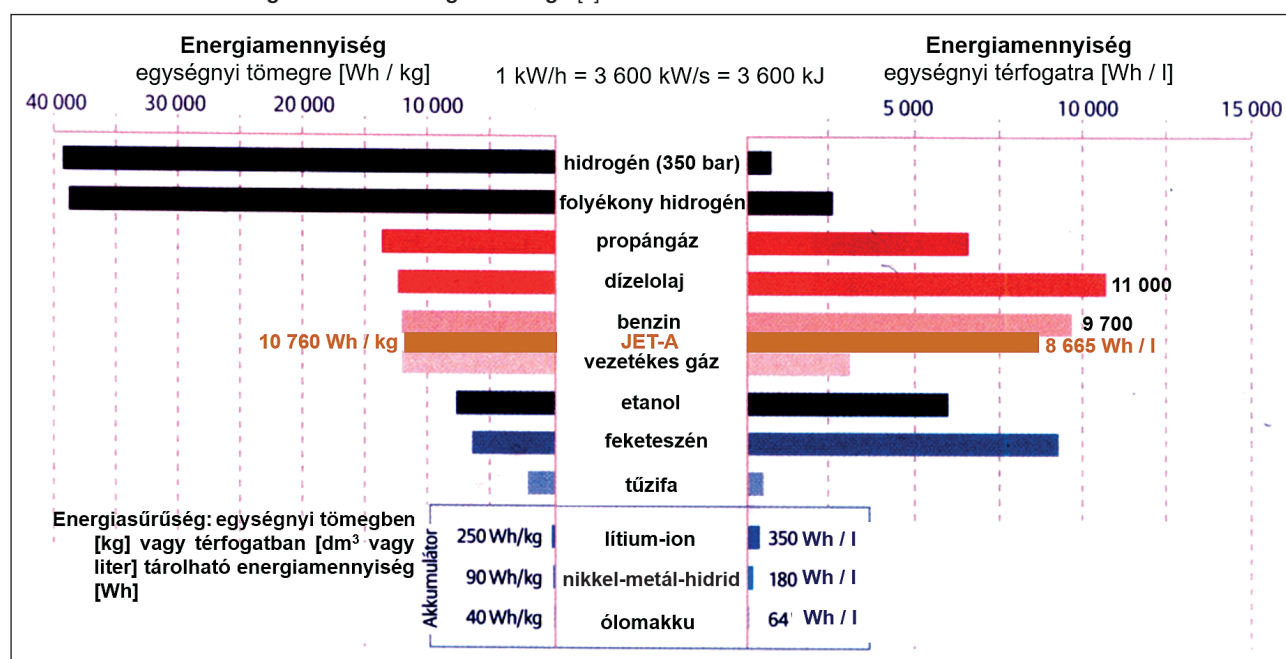
28. ábra. Különböző energiahordozók energiasűrűsége [1]
