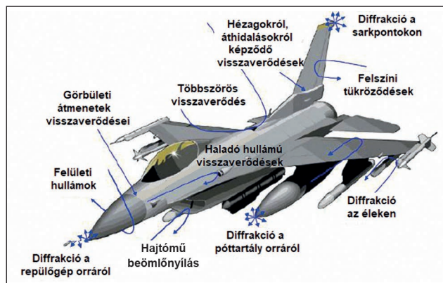
9. ábra. A radarimpulzus céltárgyról való visszaverődésének komplexitása [12]
