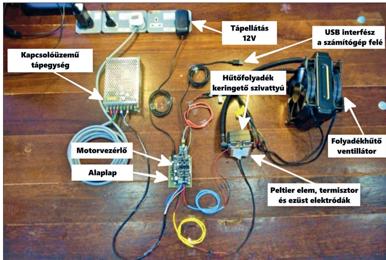
22. ábra. A termikus elven működő ízezésmanipuláló eszköz felépítése [40; 72. o.]
