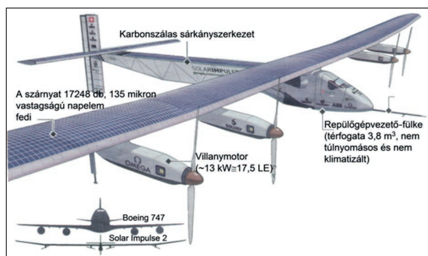
36. ábra. Solar Impulse 2 kísérleti napelemes repülőgép [6]
