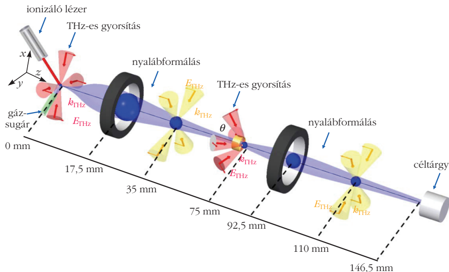
1. ábra. A THz-es impulzusokkal hajtott kompakt elektrongyorsító berendezés elvi vázlata kék színnel feltüntetve az elektronnyalábot.
