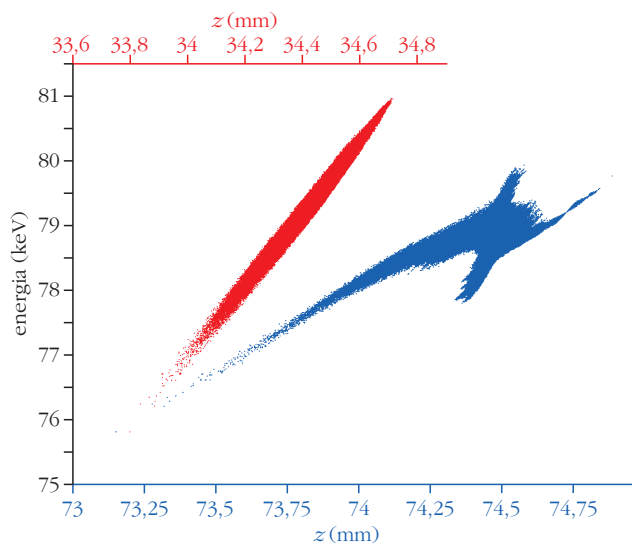
2. ábra. Az elektroncsomó energiájának longitudinális eloszlása a longitudinális kompresszió előtt (piros, felső skála), illetve a közvetlenül az utógyorsítóba való belépés előtt (kék, alsó skála).
