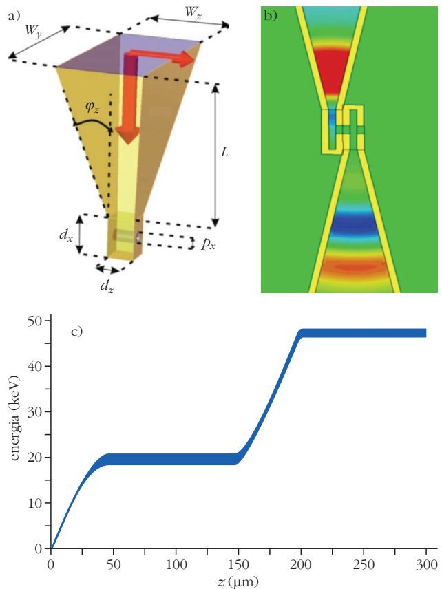
4. ábra. Kürtösterű hullámvezető elektrongyorsító és annak jellemző paraméterei (a). A két kürtőből álló gyorsító feltüntetve egy adott pillanatra a gyorsító THz-es impulzusok elektromos tereit is (b). Az elektronenergia távolsággal való növekedése (c).
