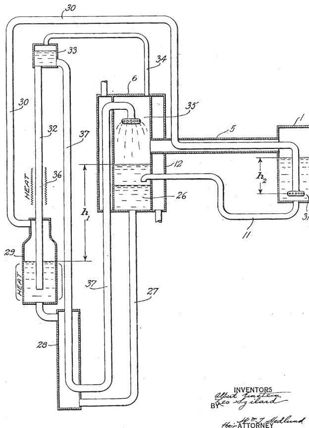
1. ábra. Einstein és Szilárd abszorpciós hűtőszekrénye az amerikai szabadalmi leírásból.
