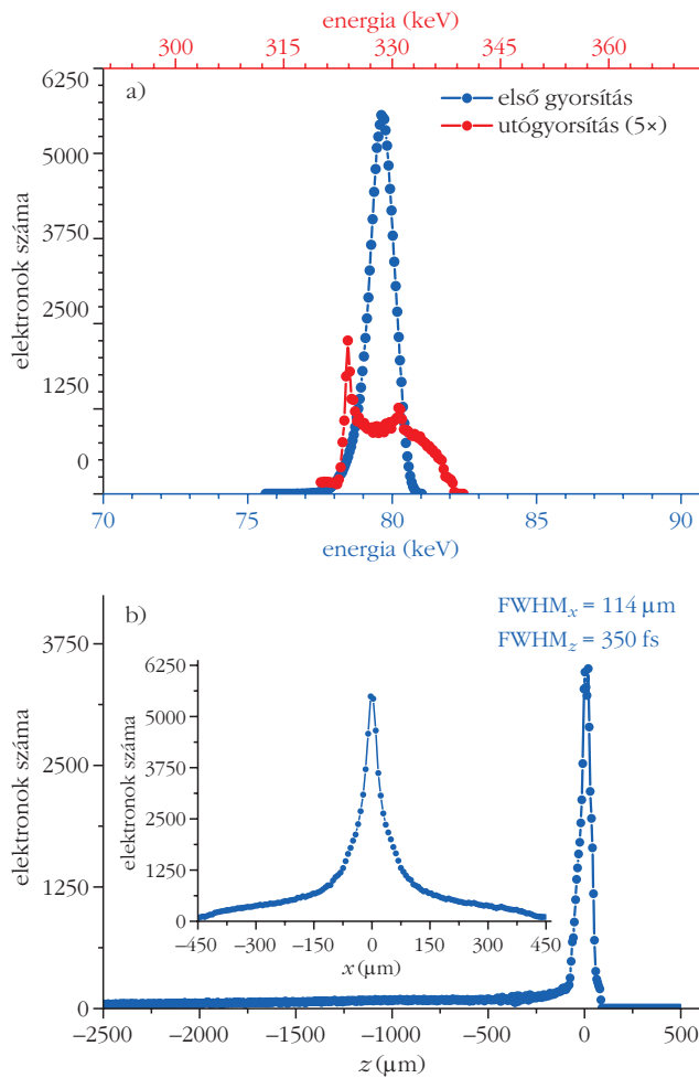
3. ábra. Az energiaspektrum az első, illetve a második gyorsító fokozat után (a). Az elektroncsomó longitudinális eloszlása a felhasználás (célterg) helyén (b). A betét a transzverzális eloszlást mutatja.
