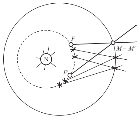
7. ábra. A Mars pályájának szerkesztése a földpálya és a marsi keringési idő ismeretében.
