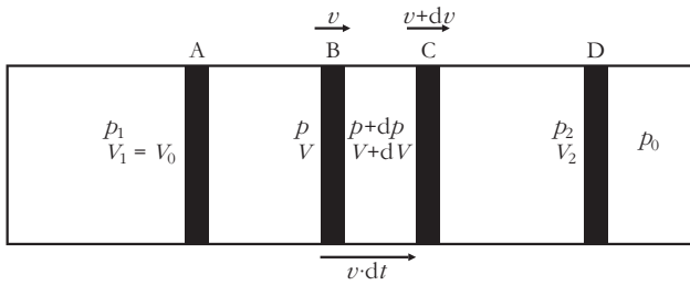
1. ábra. Hőszigetelt hengerben hőszigetelt dugattyú ideális gázt zár el. A dugattyú „A” helyzete tartozik a kiinduló állapothoz, a „B” egy tetszőleges állapothoz, a „C” egy annál dt idővel későbbi állapothoz, a „D” pedig az első megálláshoz.
