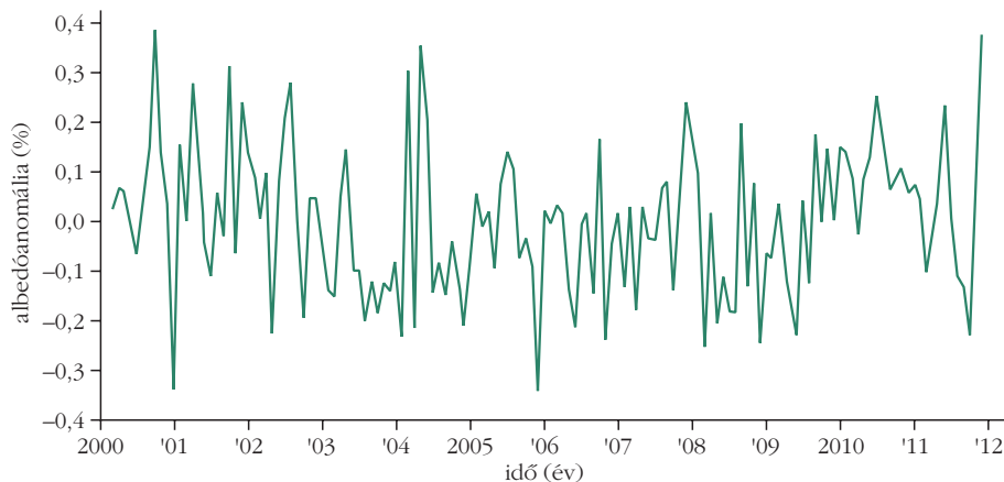
4. ábra. A százalékban mért planetárisalbedó-anomália időbeli változása [6].
