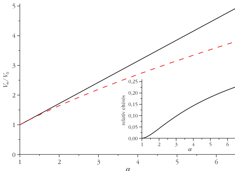
4. ábra. A vég- és a kezdőállapot térfogataránya \alpha függvényében. A folytonos görbe a (17) összefüggés alapján, a szaggatott a Poisson-törvénnyel történő számolás eredménye. A betét a relatív eltérést mutatja \alpha függvényében.
