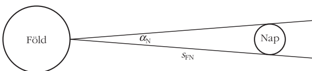
5. ábra. A Nap mérete látószög alapján, a Föld–Nap távolság ismeretében.
