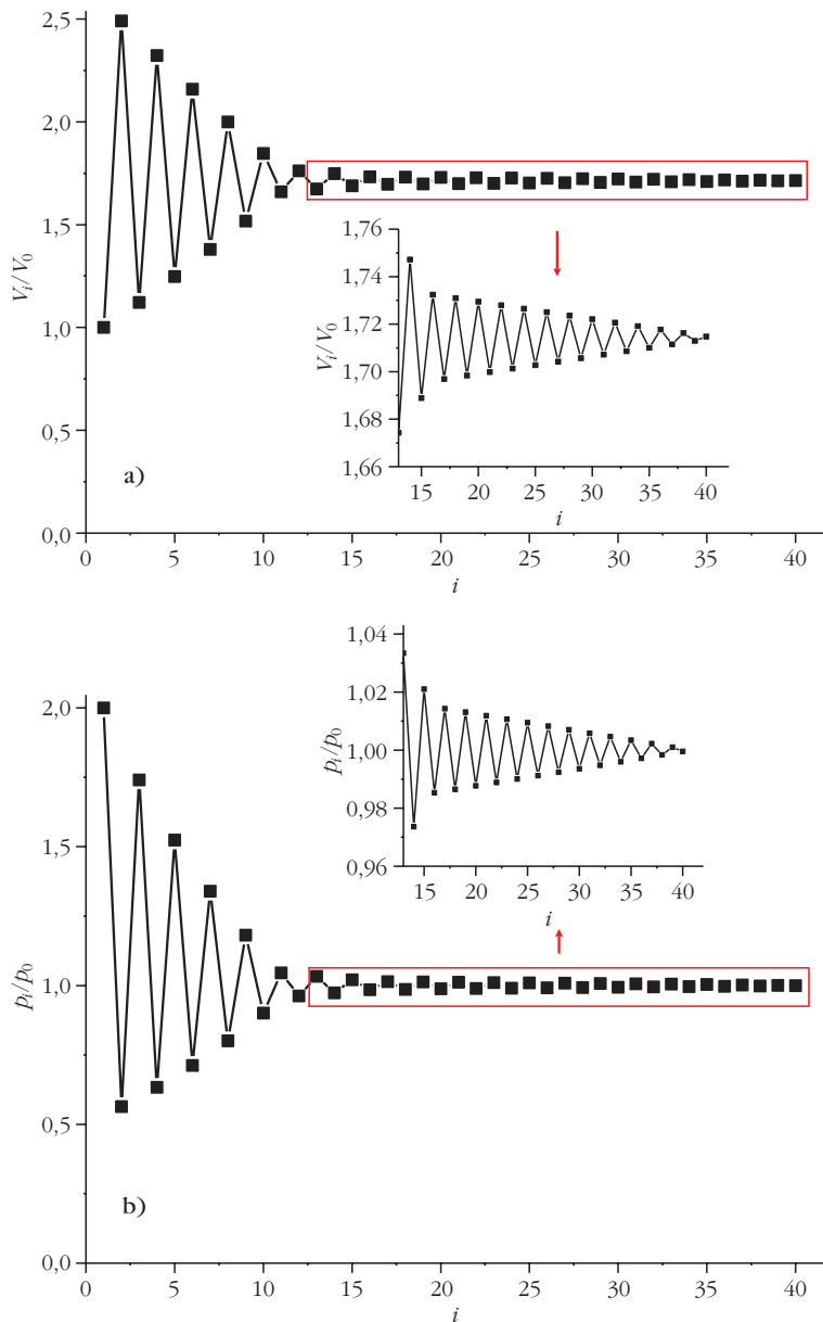
3. ábra. A dugattyú fordulópontjaihoz tartozó (a) térfogat-, illetve (b) nyomásértékek V_0 , illetve p_0 egységeiben \alpha = p_1/p_0 = 2 értéket feltételezve, az egymást követő fordulópontok számának függvényében (a \beta = p_s/p_0 paraméter a szimuláció során változik). A betéttábrakon a 13. fordulópontot követő folyamat felnagyítva látható.
