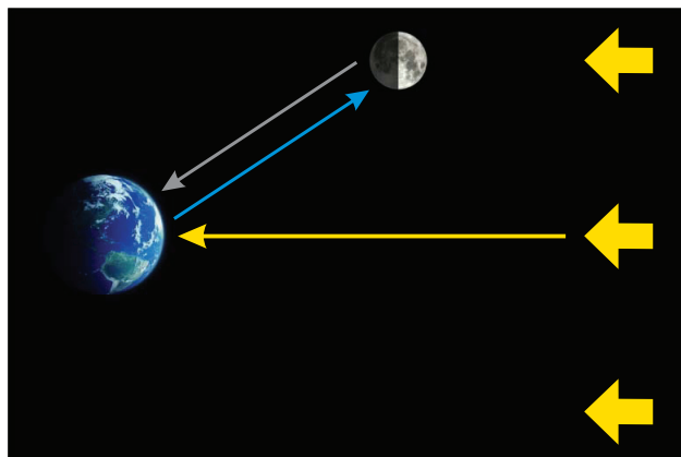
1. ábra. A földfény kialakulásának elve [3]. A Hold „égi tükörként” veri vissza a Földre a Föld által odatükrözött napfényt.
