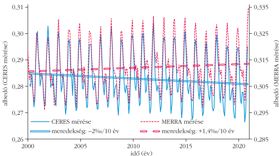
2. ábra. A CERES (folytonos görbe) és MERRA (szaggatott görbe) albedóadatok és trendjük (dupla görbék) 2000 és 2020 között [5]. A CERES szerint 10 év alatt mintegy 2‰-al csökken, míg a MERRA adatai szerint 1,4‰-al nő az albedó.
