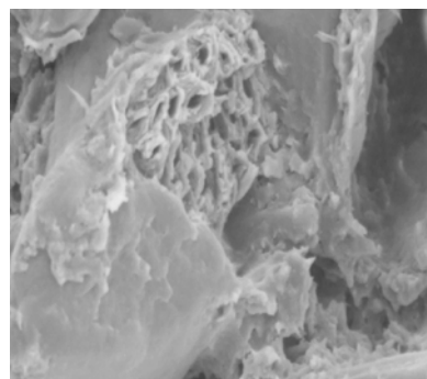
6. ábra – Törési felület kiváló rost-mátrix kapcsolat
