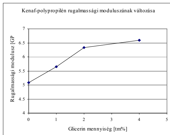
3. ábra – a kenaf-polipropilén kompozit hajlítórugalmassági moduluszának változása a glicerín mennyiség függvényében
