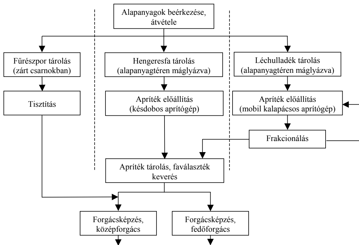
2. ábra – A vizsgált technológia folyamatábrája
