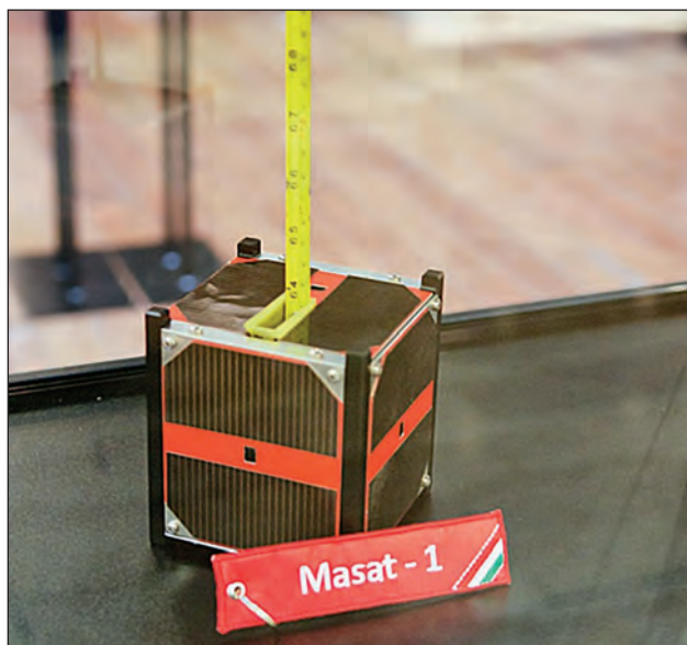
1. ábra. Az első magyar műhold. Mérete a cubesat-ok alapegysége, a 10 cm élhosszúságú kocka
