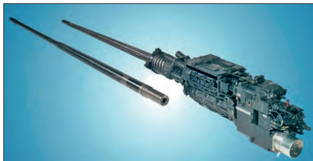
3. ábra. Az MK 35/50 Rh 503 típusú gépágyú (Fotó: Rheinmetall)
