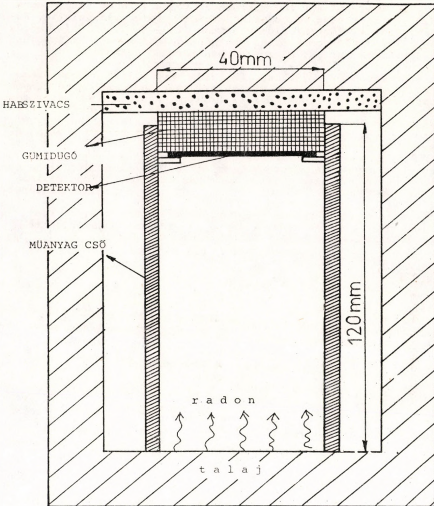
TERMÉSZETES RÁDIOAKTIVITÁS MÉRÉSE A TALAJBAN NYOMDETEKTORRAL
