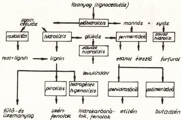
1. ábra: A faanyag vegyipari felhasználási lehetőségei /Chornet, 1979./
