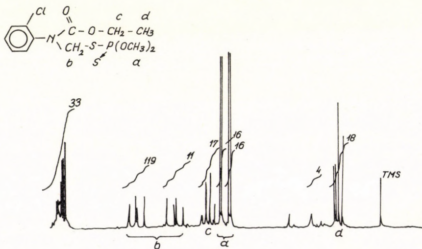
Az O,O-dimetil-S-/N-/2-klór)fenil)-etil-karbamát/ metil-ditiofoszfát ^1\text{H} spektruma
