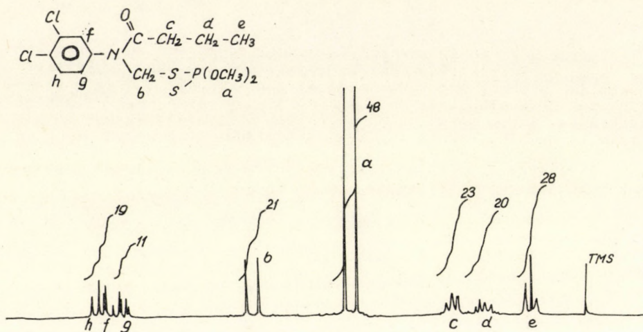
Az O,O-dimetil-S-/N-/3,4-diklórfenil-/butirilamino/ metil-ditiofoszfát ^1\text{H} spektruma
