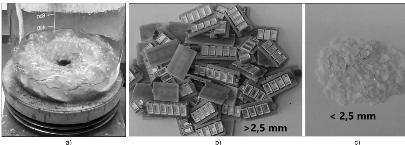
■ 3. ábra. A lúgos feltáró oldás (a) és termékei, a fémes maradvány (b) és a fényporos magok (c)
