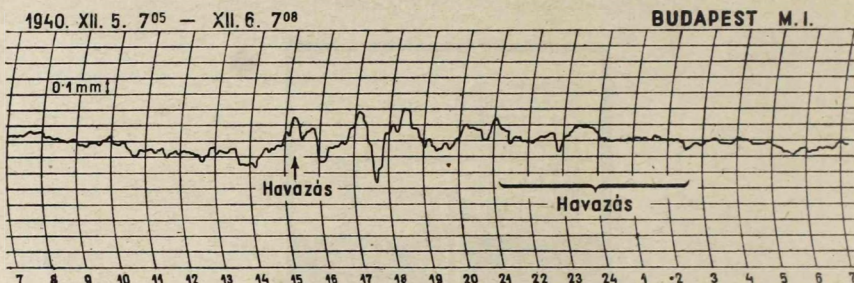
2. ábra. Mikrobarográf görbéje felsikló (meleg) front alkalmával.
