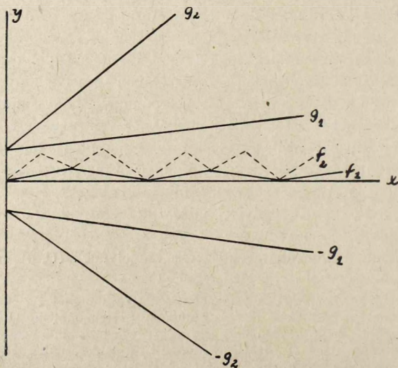
15. ábra. A síkgörbék ívhossza.
