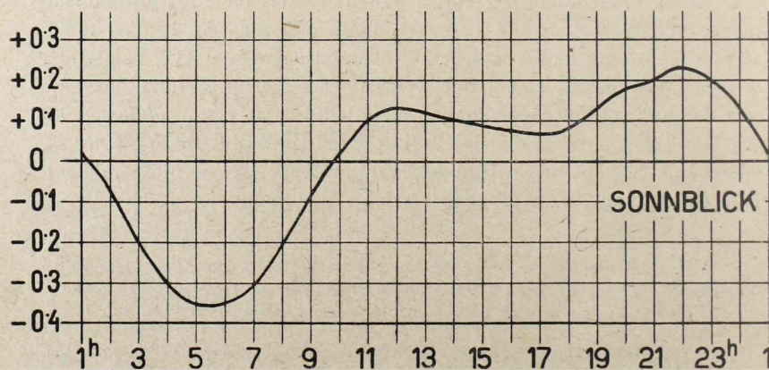
4. ábra. A légnyomás napi menete: 120 m (Ógyalla), 1000 m (Kékestető) és 3000 m (Sonnblick) magasságban.
