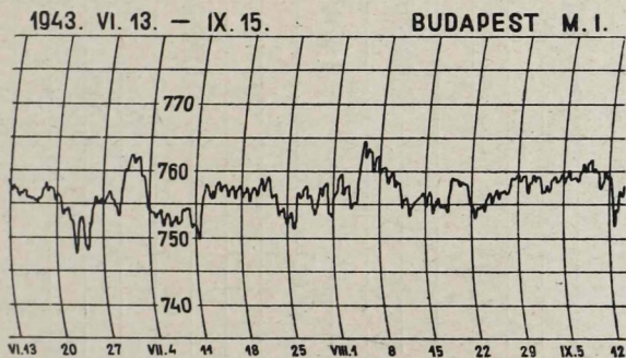
6. ábra. Makrobarográf görbéje a nyár folyamán.
