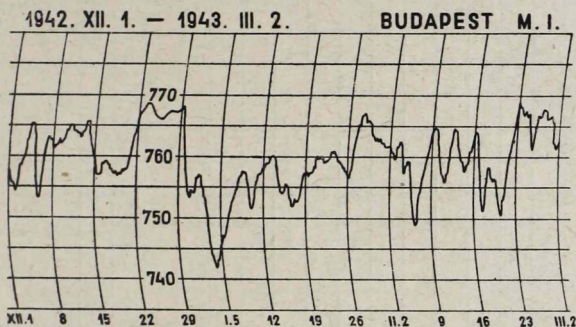
5. ábra. Makrobarográf görbéje a tél folyamán.
