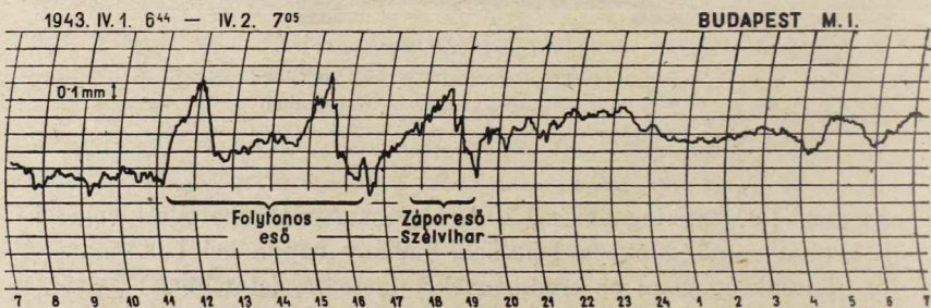
3. ábra. Mikrobarográf görbéje betörési (hideg) front alkalmával.
