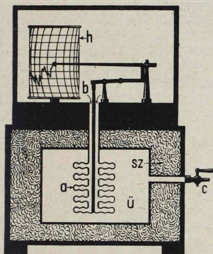
1. ábra. Mikrobarográf vázlatos rajza.
