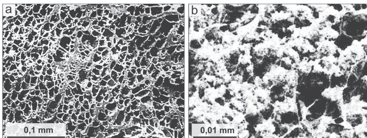
1. ábra. Biopolimer mátrix és a kicsapódott karbonátásványok szöveti kapcsolata recens sztromatolítból vett mintán (DEFARGE et al. 1996. krio-SEM-felvétel alapján FotoSketcher programmal készített rajz)
