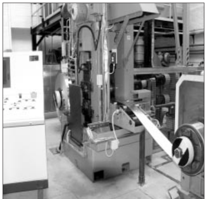
5. ábra: VON ROLL kísérleti hengerállvány
