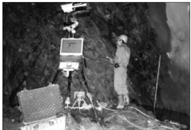
10. ábra: Vágat geotechnikai dokumentálás
