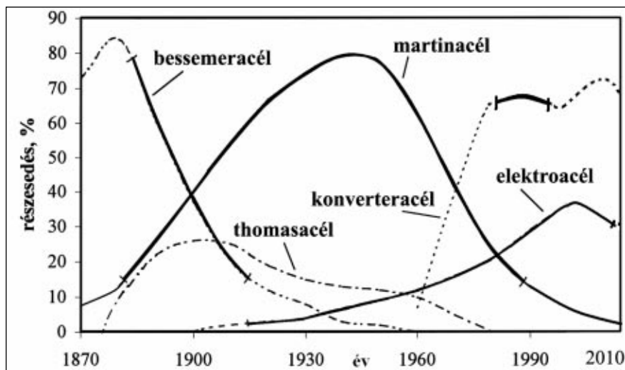
1. ábra: Az acélgártó eljárások életgörbéi
