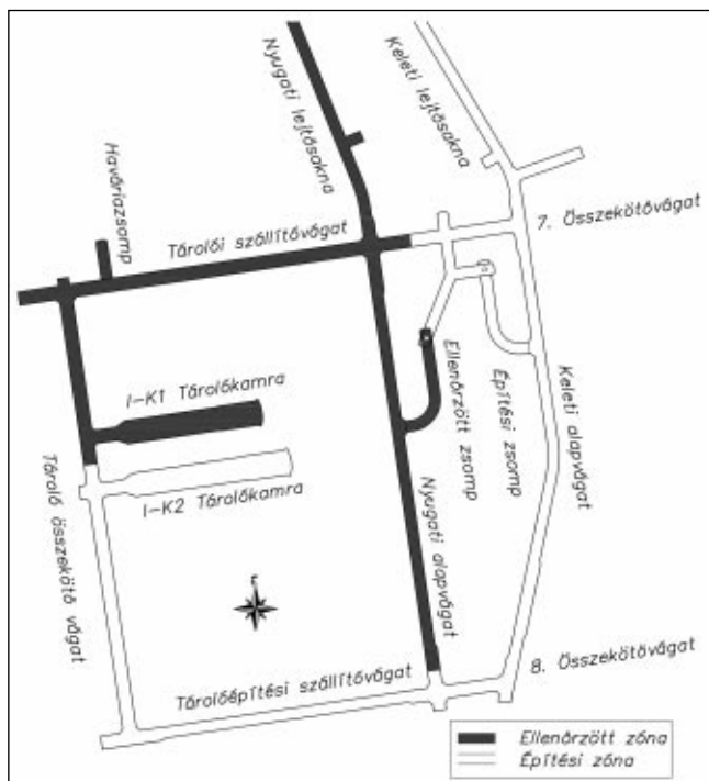
5. ábra: Az NRHT kamramező elrendezési rajza
