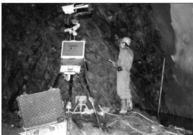
10. ábra: Vágat geotechnikai dokumentálás
