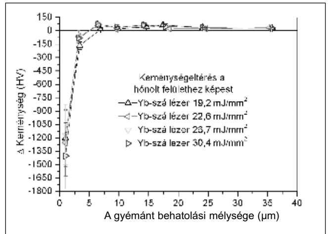
■ 9. ábra. Yb-szállézerrel kezelt mintasorozat (a)–d) minták keménységértékeiből kivonva a hőnolt felület keménységértékei
