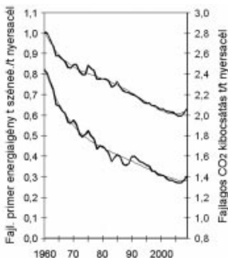
7. ábra: Az acélgártás energiaterjesztésének és CO 2 -kibocsátásának változása Németországban 1960 óta
