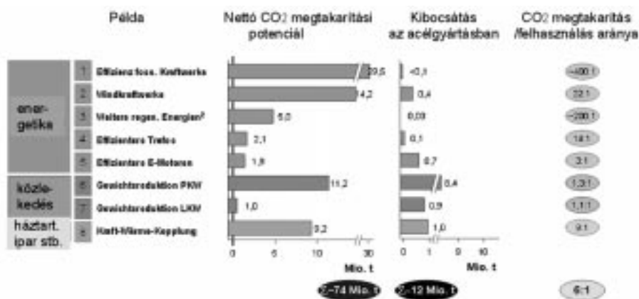
8. ábra: Az acél innovatív alkalmazásával hatszor annyi széndioxid-kibocsátás takarítható meg, mint amennyi az acéltermelésben keletkezik (1. hatásfok fosszilis erőmű esetén, 2. szélenergia, 3. további megújuló energiák, 4. hatékonyabb transzformátorok, 5. hatékonyabb elektromotorok, 6. súlycsökkentés teherautóknál, 7. súlycsökkentés személyautóknál, 8. kapcsolt erőművek)
