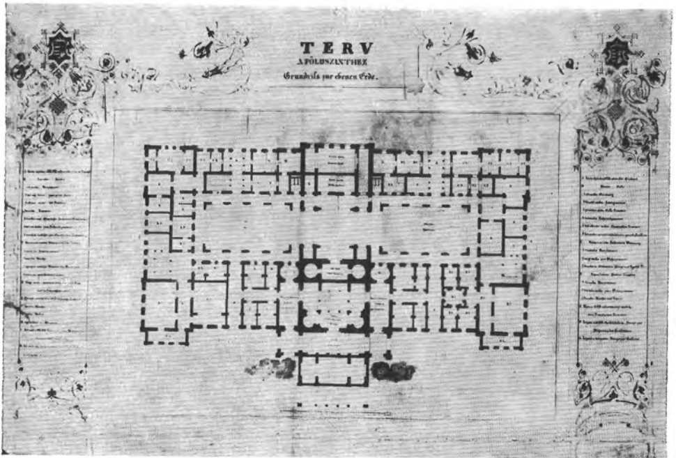
4. Feszl Frigyes Országház-terve. Földszint alaprajza.
