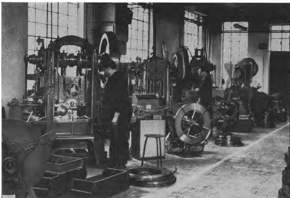
3. Egyszerű lakatlevágó automata gépcsoport, 1938.
