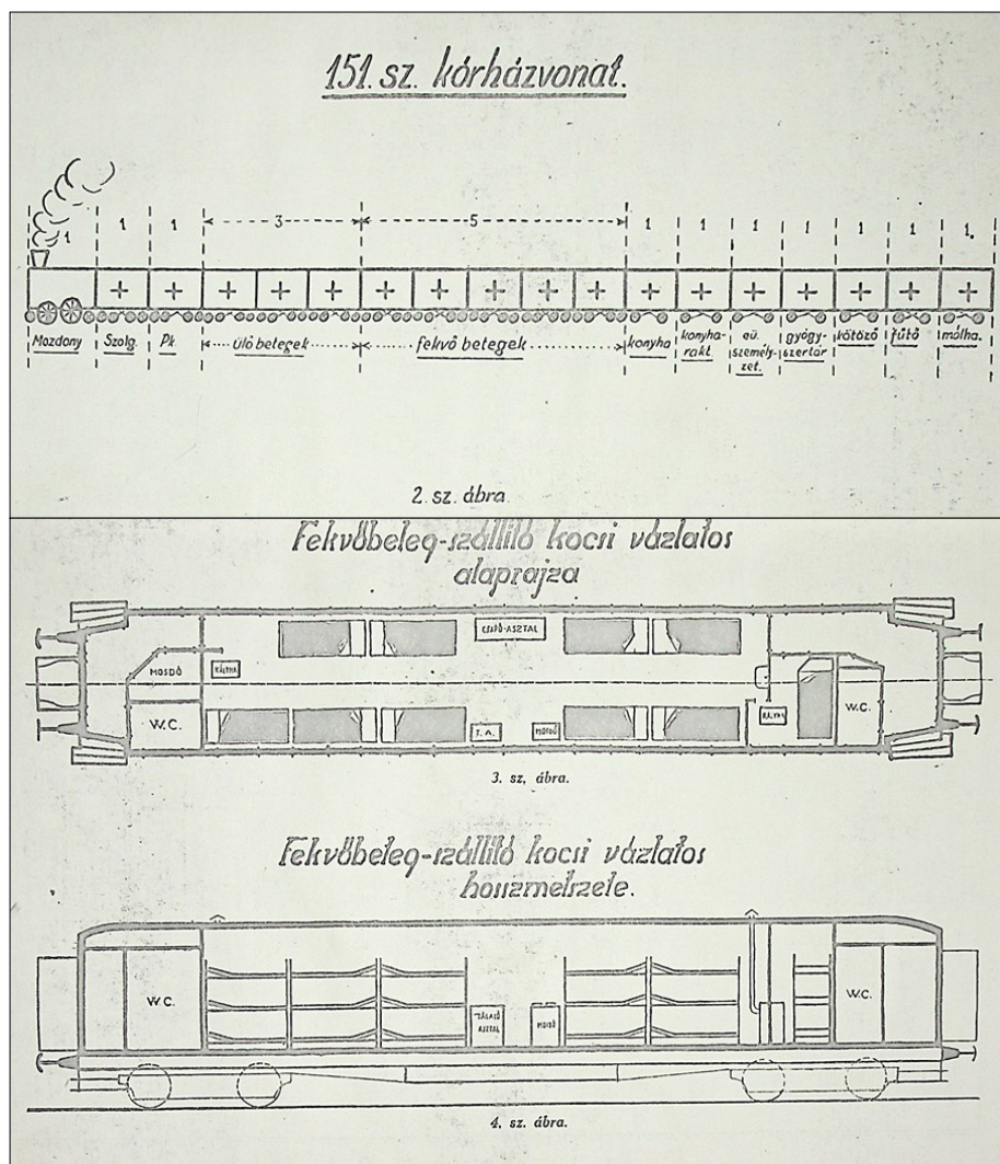
A 151-es kórházvonat rajza a Honvédorvos 1942. évi 1. számában p. 6-7.
