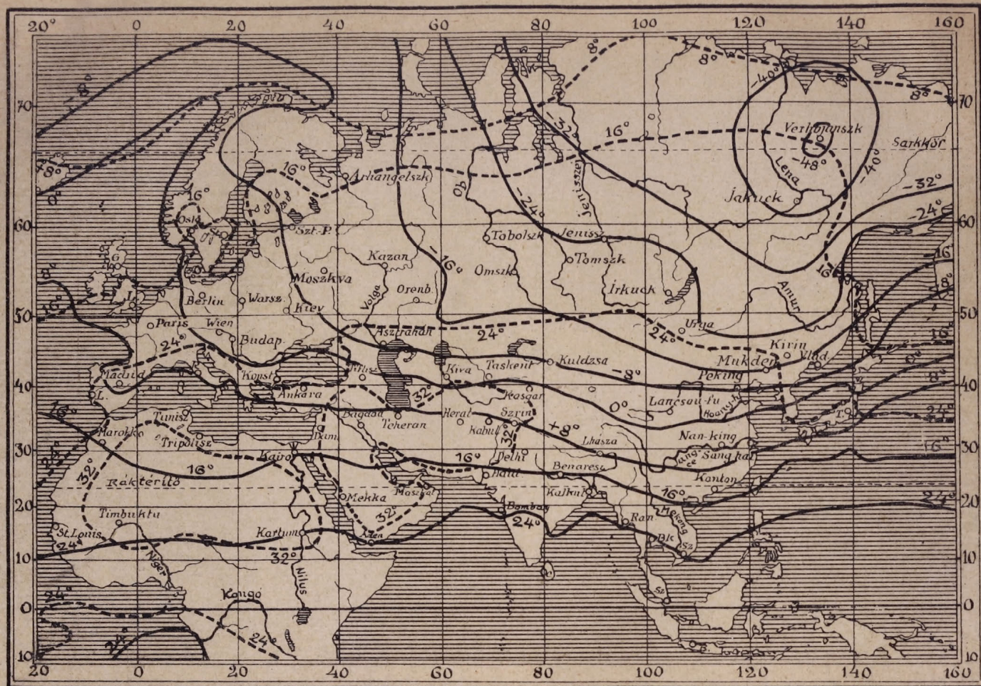
12. ábra. A hőmérséklet eloszlása Euráziában. A teljesen kihúzott vonalak a januáriusi, a szaggatott vonalak a júliusi izotermák.
