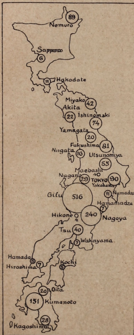
3. ábra. A földrengések átlagos évi száma Japán egyes földrengés-megfigyelő állomásán. A számok a főljegyzett földrengések számai, a körök nagysága arányos ezekkel a számokkal.
