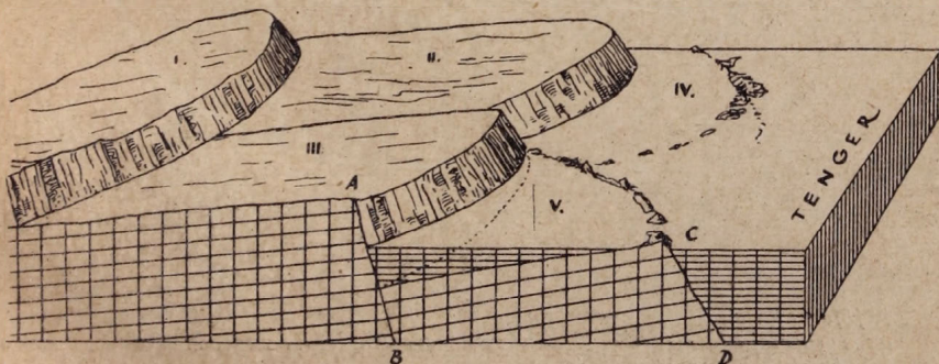
2. ábra. A keletázsiai szigetívek és felvetődések szerkezete. AB, CD vetődések, I—V. felvetődött kéregdarabok.
